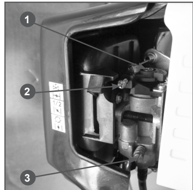
Рис. 14 Расположение винтов регулировки карбюратора.
